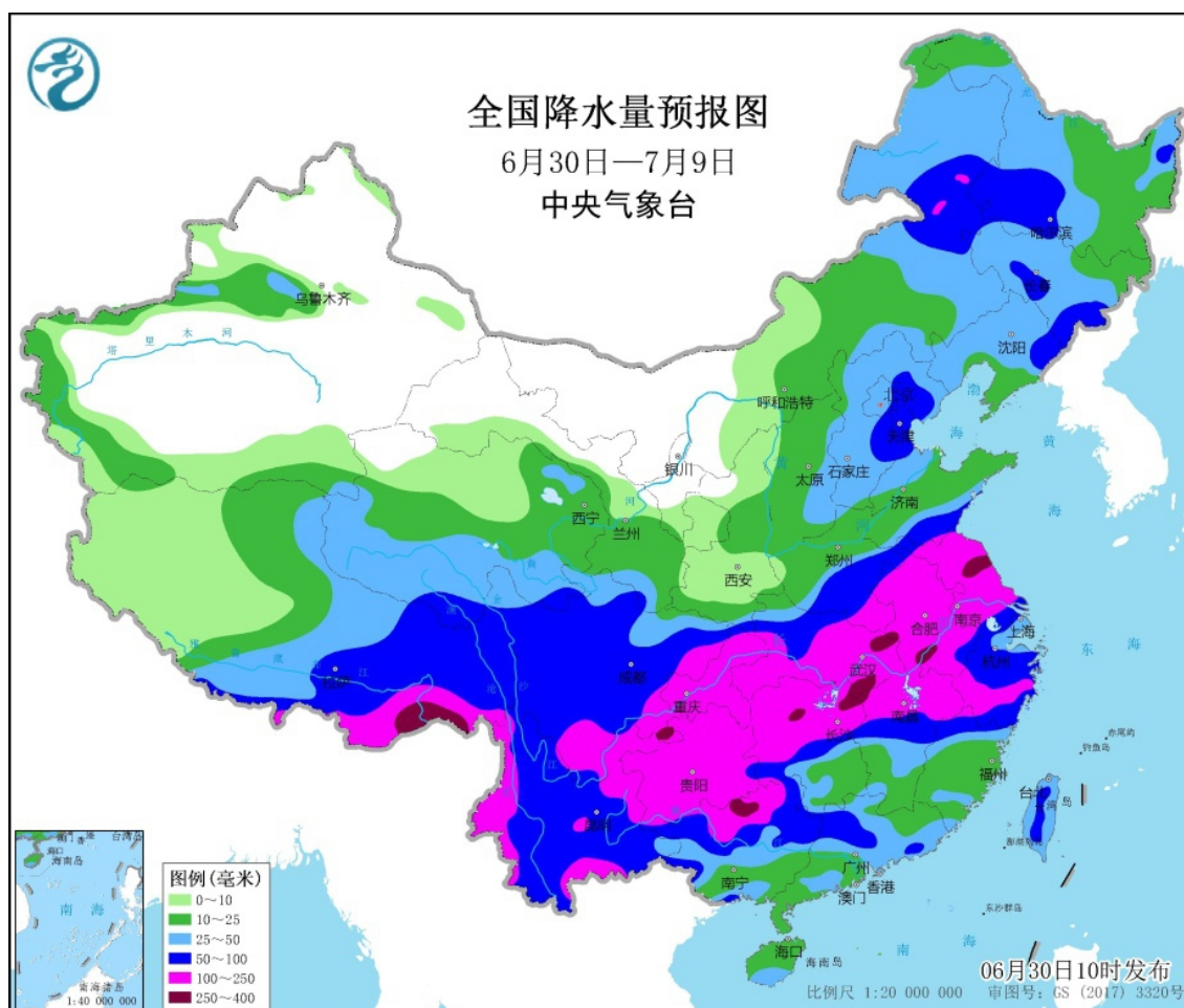
图 1 6 月 30 日到 7 月 9 日全国降水量预报图
