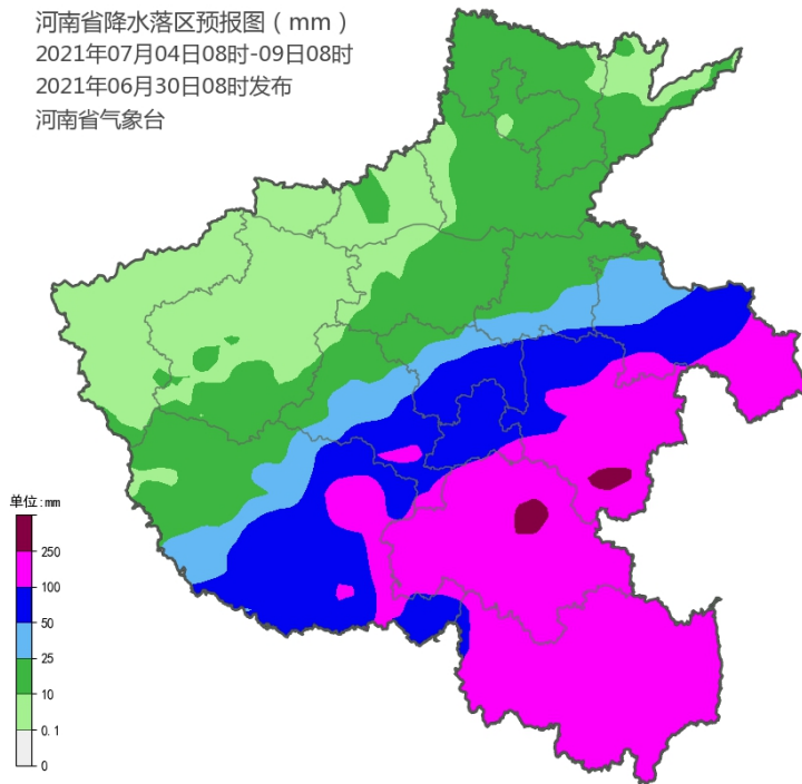
图 3 7 月 4 日 08 时-9 日 08 时河南省降水量预报
