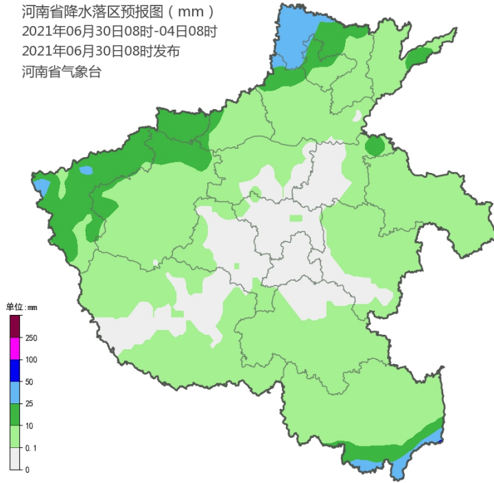
图 2 6 月 30 日 08 时-7 月 4 日 08 时河南省降水量预报
